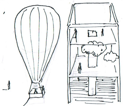
ATMOSFERA
