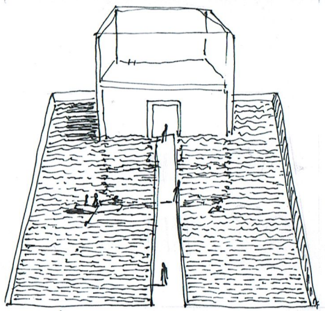
HIDROSFERA
