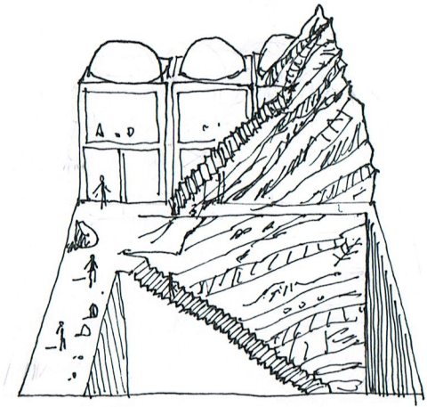
LITOSFERA
